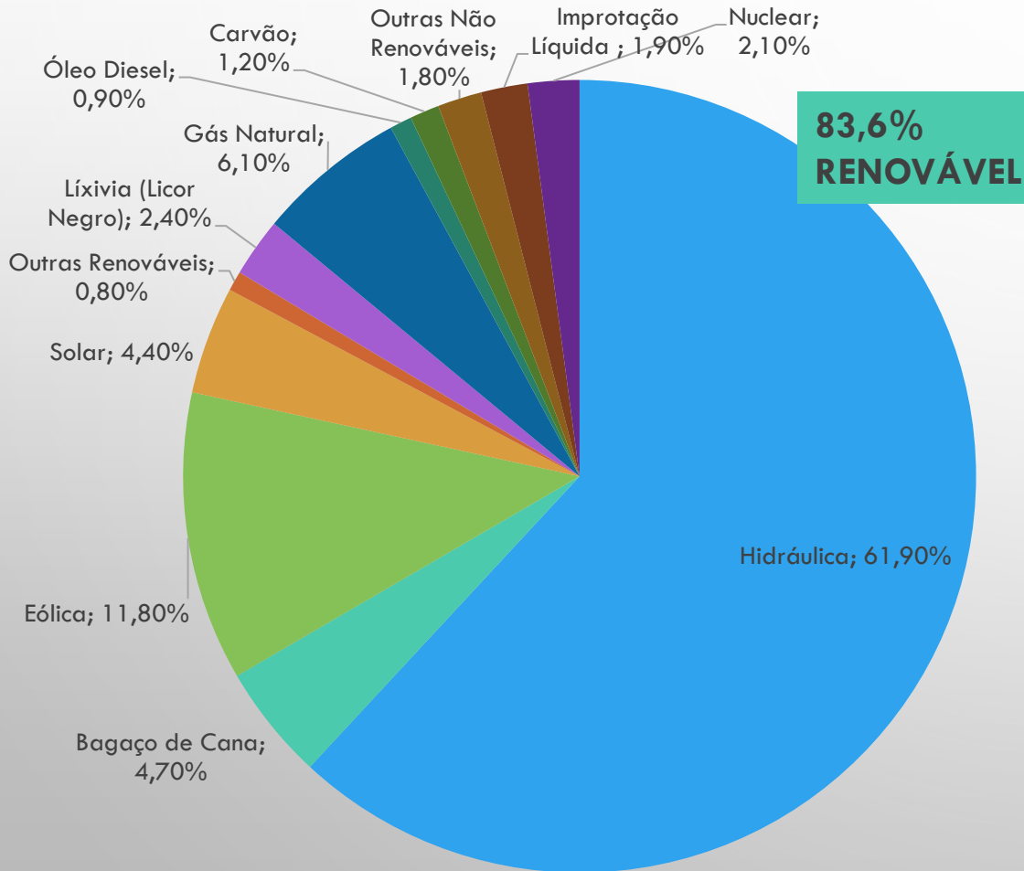
MATRIZ ELÉTRICA 2022
