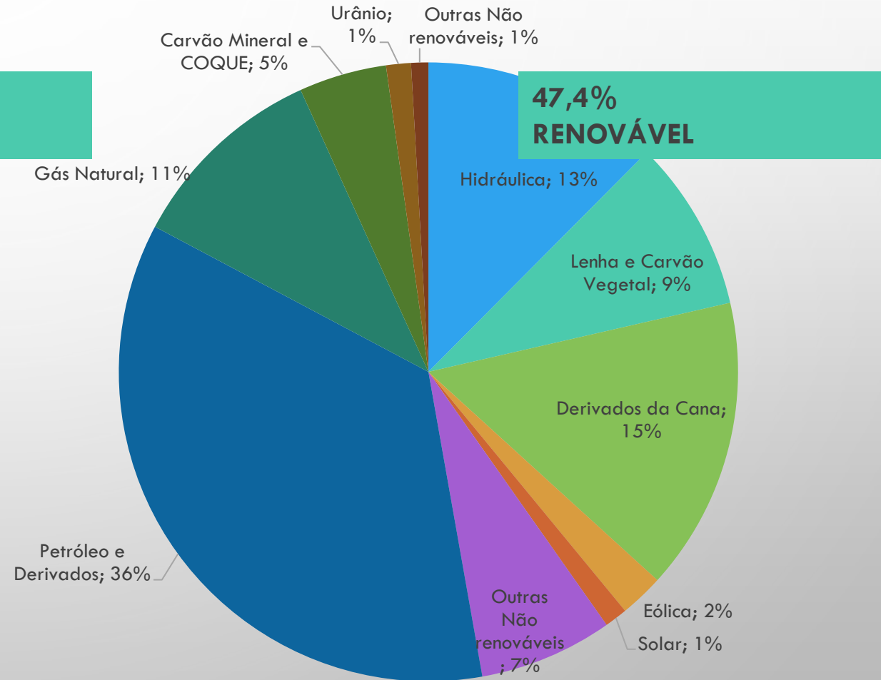
MATRIZ ENERGÉTICA 2022
